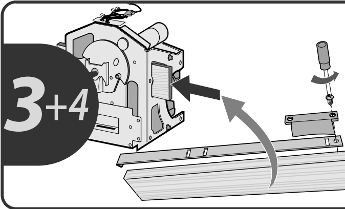
动力组安装
