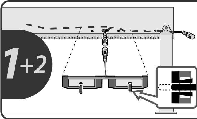
轨道安装
